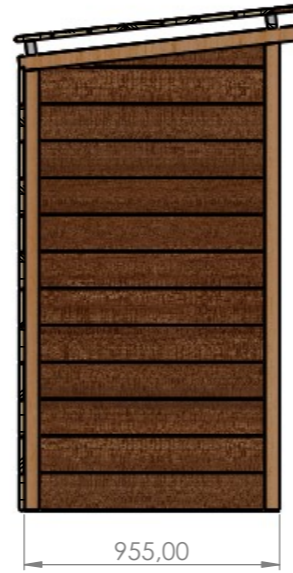
SEZIONE A-A
