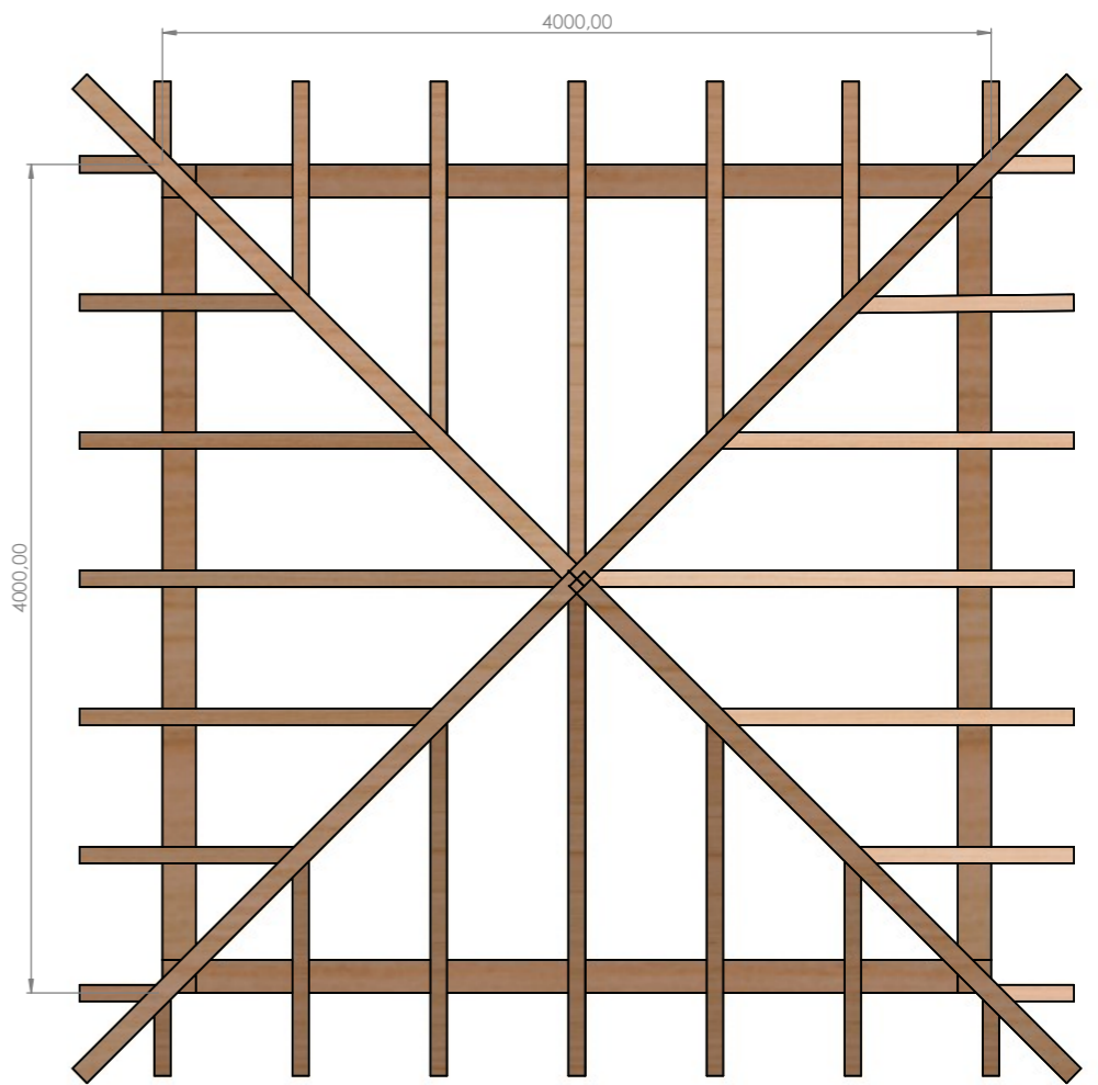
VISTA STRUTTURA TETTO
