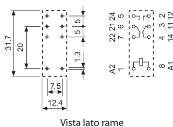
Vista lato rame
