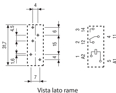
Vista lato rame
