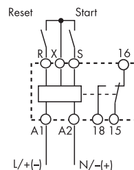
Schema di collegamento (con START esterno)
