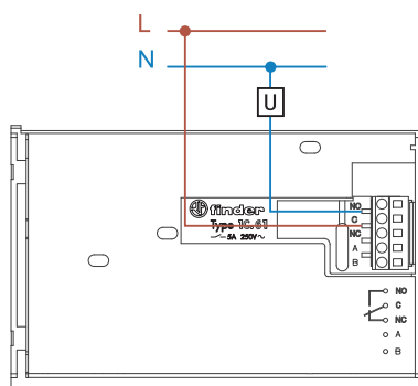
Schema elettrico
