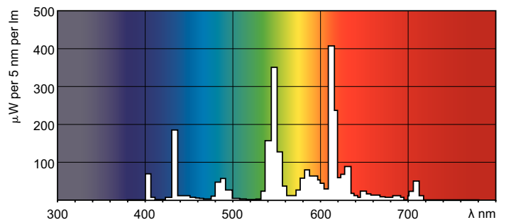
Designazione colore /830
