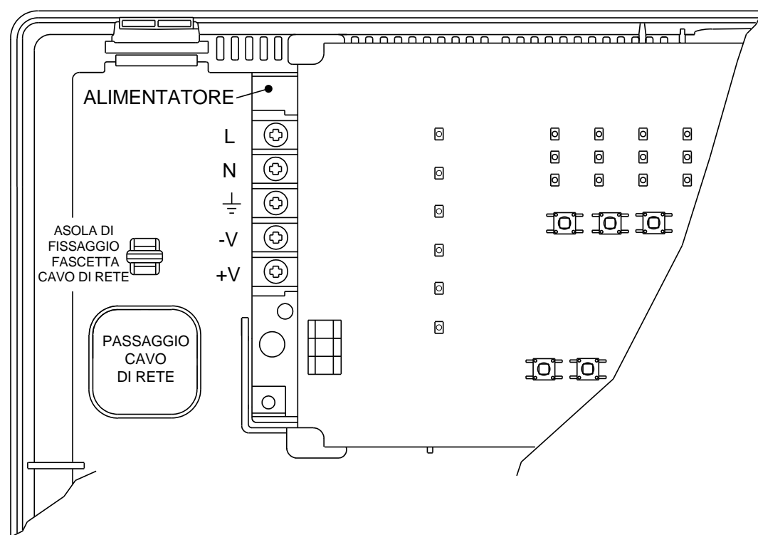
Figura 1 - Morsettiera alimentatore
