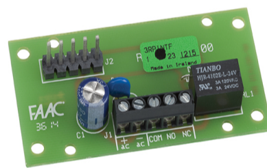
Interfaccia Relè per l'utilizzo di riceventi RP per collegamenti filari
