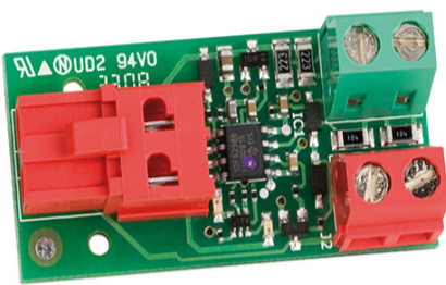
Interfaccia BUS XIB (per scheda E045 o E045S o E024S con fotocellula no BUS)
