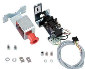
XB LOCK blocco motore bistabile A1000 c/pomello
