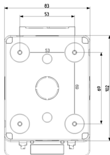
Vista posteriore
